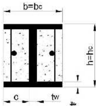
Fig. 7.6.1 - Rapporti dimensionali
