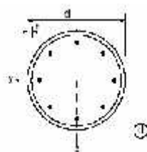
Figura 4.3.7 - Sezione tipo di colonna composta circolare riempita di calcestruzzo in cui è possibile considerare il confinamento del calcestruzzo
