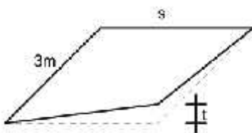
Fig. 5.2.14 - Sghembo ammissibile
