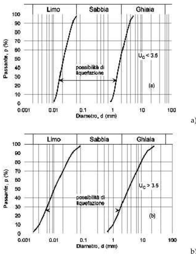
Fig. 7.11.1 – Fusi granulometrici di terreni suscettibili di liquefazione
