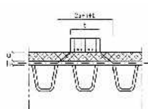
Fig. 5.1.3b - Diffusione dei carichi concentrati negli impalcato a piastra ortotropa
