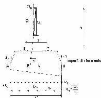
Fig. 5.2.5 - Distribuzione trasversale in rettifilo delle azioni per mezzo delle traverse e del ballast. In figura, Q_h rappresenta la forza centrifuga definita al successivo §5.2.2.3.1
