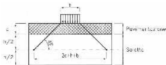
Fig. 5.1.3a - Diffusione dei carichi concentrati nelle solette
