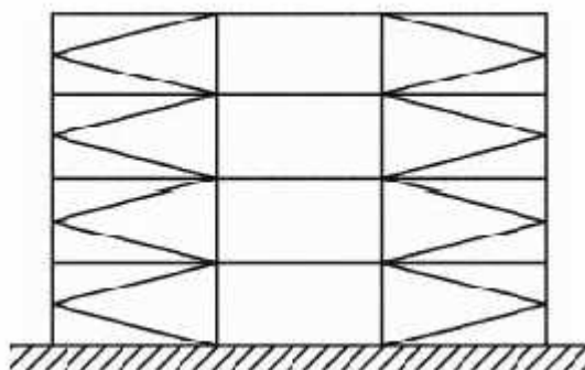
b3) Strutture con controventi concentrici a K
